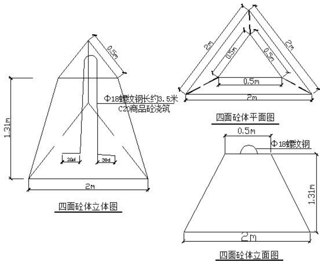
1m 3 预制C20商品砣四面体示意图
