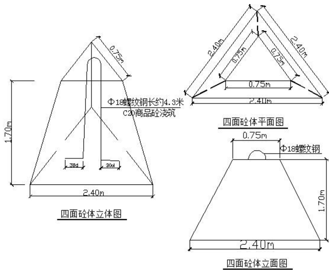
2m 3 预制C20商品砣四面体示意图
