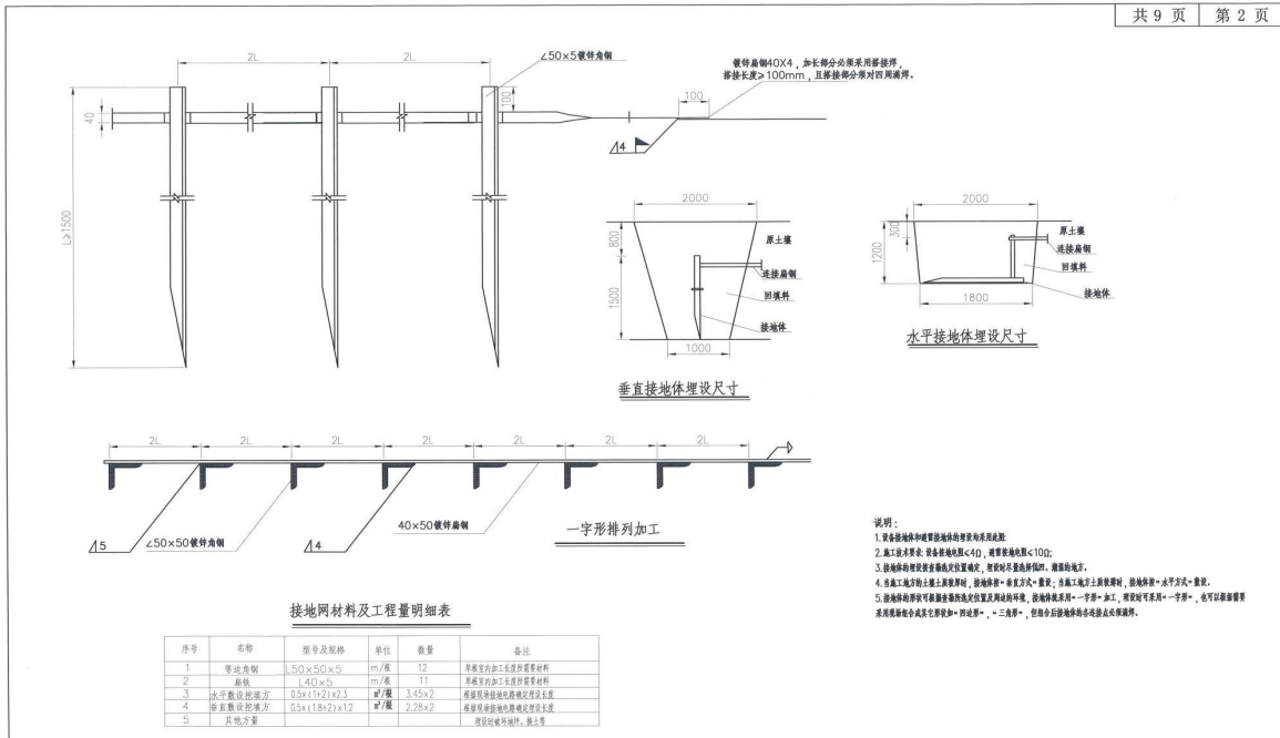
附图 5：防雷接地制作示意图
